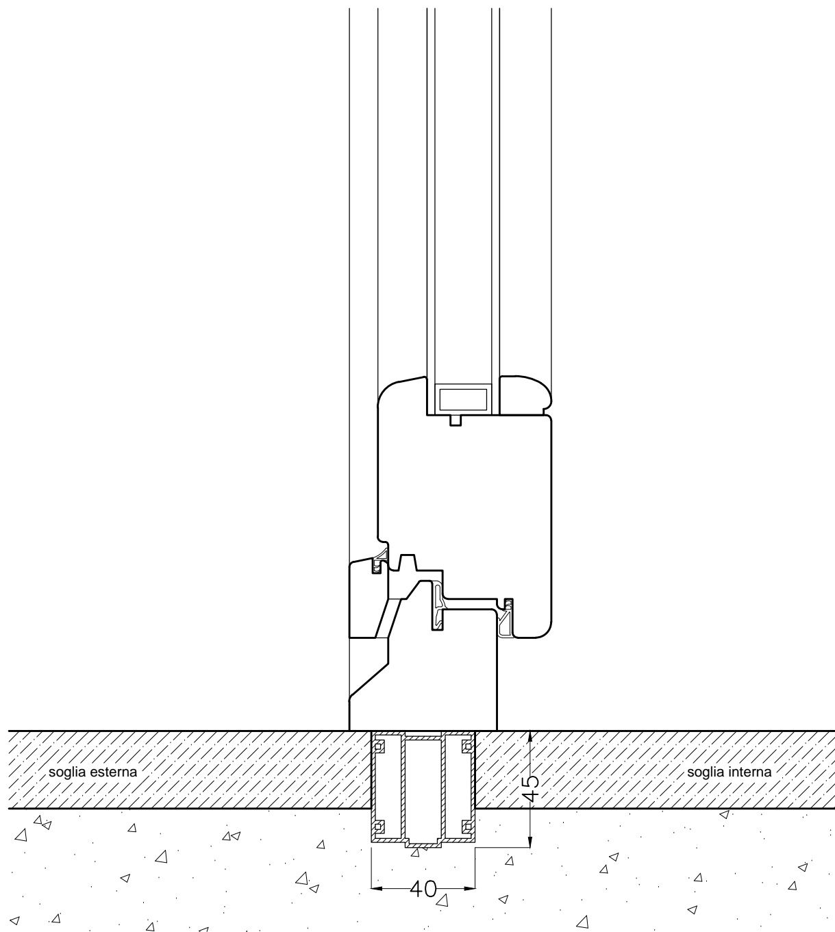
BARRIERA TERMICA A FILO SOGLIA sezione finestra
